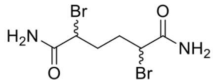
2,5-Dibromohexanediamide ( 2 )
